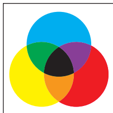
▲図1 色の三原色
