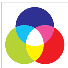
▲図1 光の三原色
